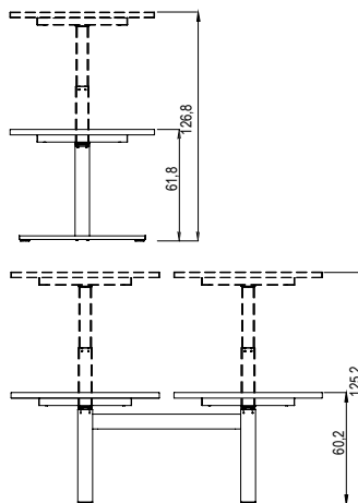
3-stage legs 3 étapes 3 Stufig
