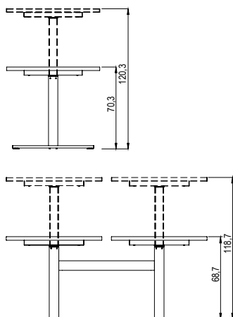
2-stage legs 2 étapes 2 Stufig
